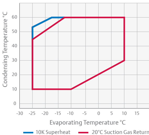
YB - R455A
