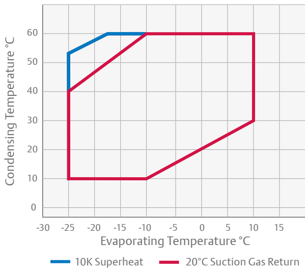
YB - R454A
