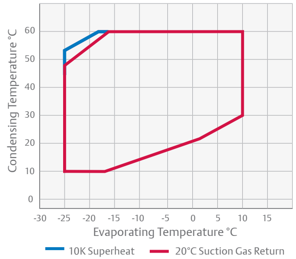
YBD - R454C
