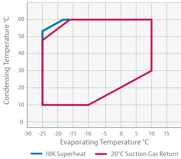
YB - R454C
